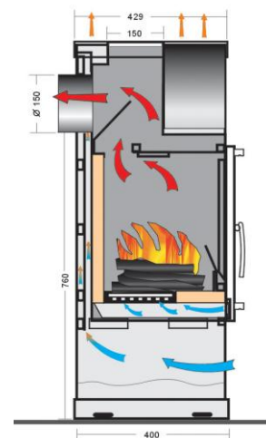
Šķēsgriezums-“Vienybė-05”
