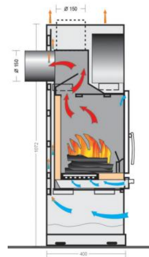
Šķēsgriezums-“Vienybė-02”
