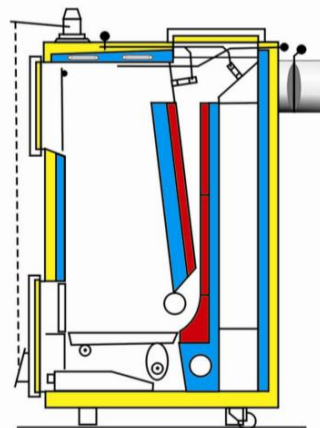
Šķērsgriezums „Vienybė-20M”
