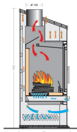
Šķēsgriezums-“Vienybė-07”
