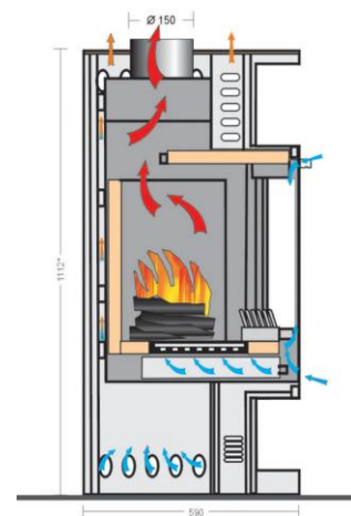
Šķēsgriezums-“Vienybė-04”
