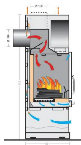
Šķērsgriezums-„Vienybė-06-6“
